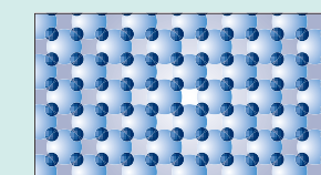
氷 (個体) の時の水分子
