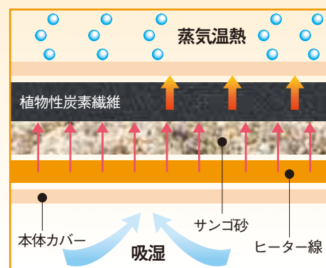
ULMO 構造図
