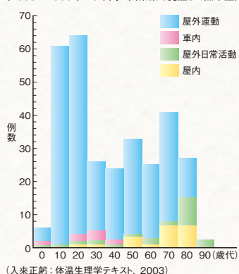
各年齢における熱中症発症数およびその原因 (1995～2000年の5年間に山梨県で発症した熱中症)
